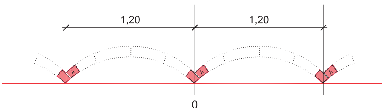
10. ábra: az „A” sarokkövek indítása
