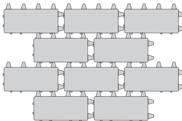
Futókötés
