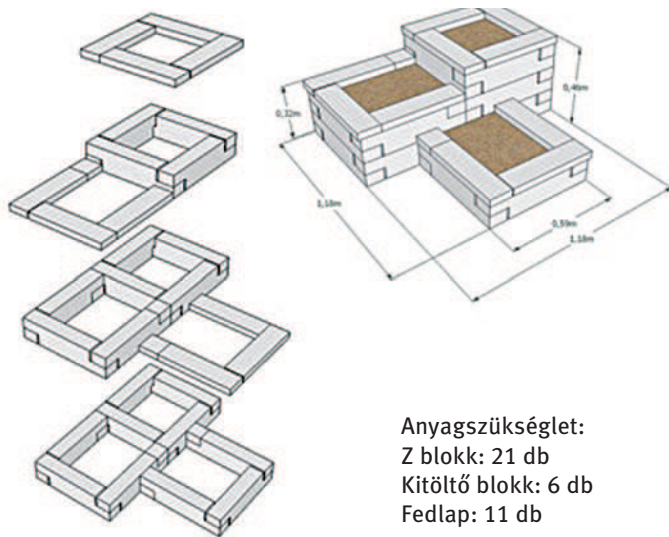
Egy 120x120x47 cm növénykazetta kialakításának vázlata
