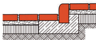
Két, nem azonos magasságú felület választóvonala, egyoldalúan lerakott szegélykövekből kialakított szegély.
